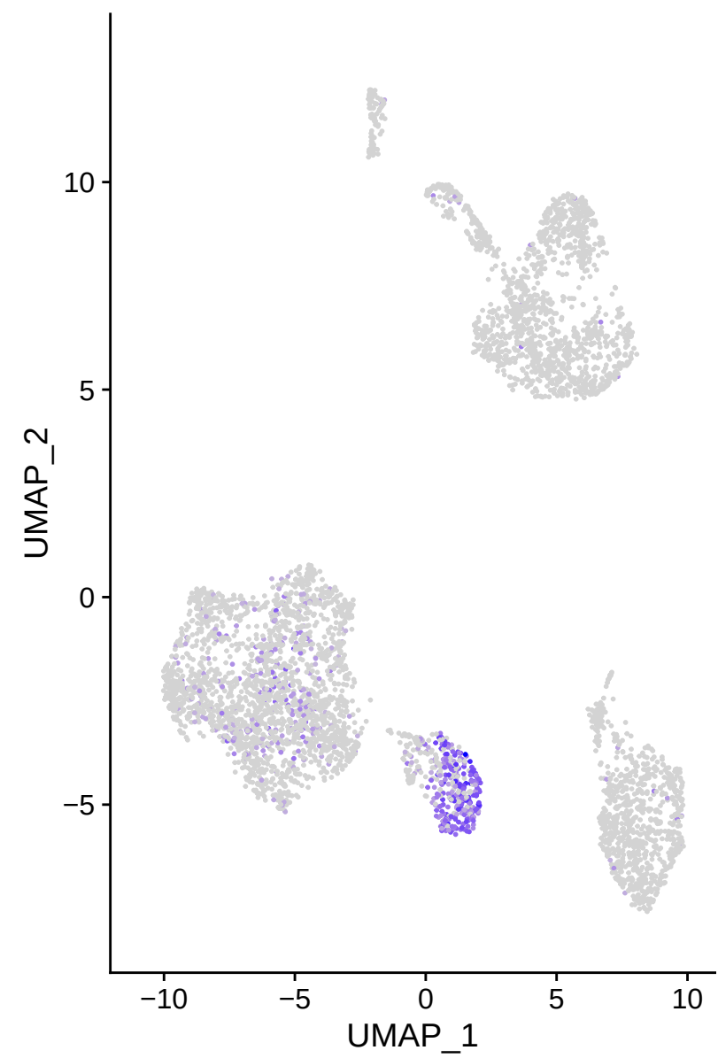
FGF4
