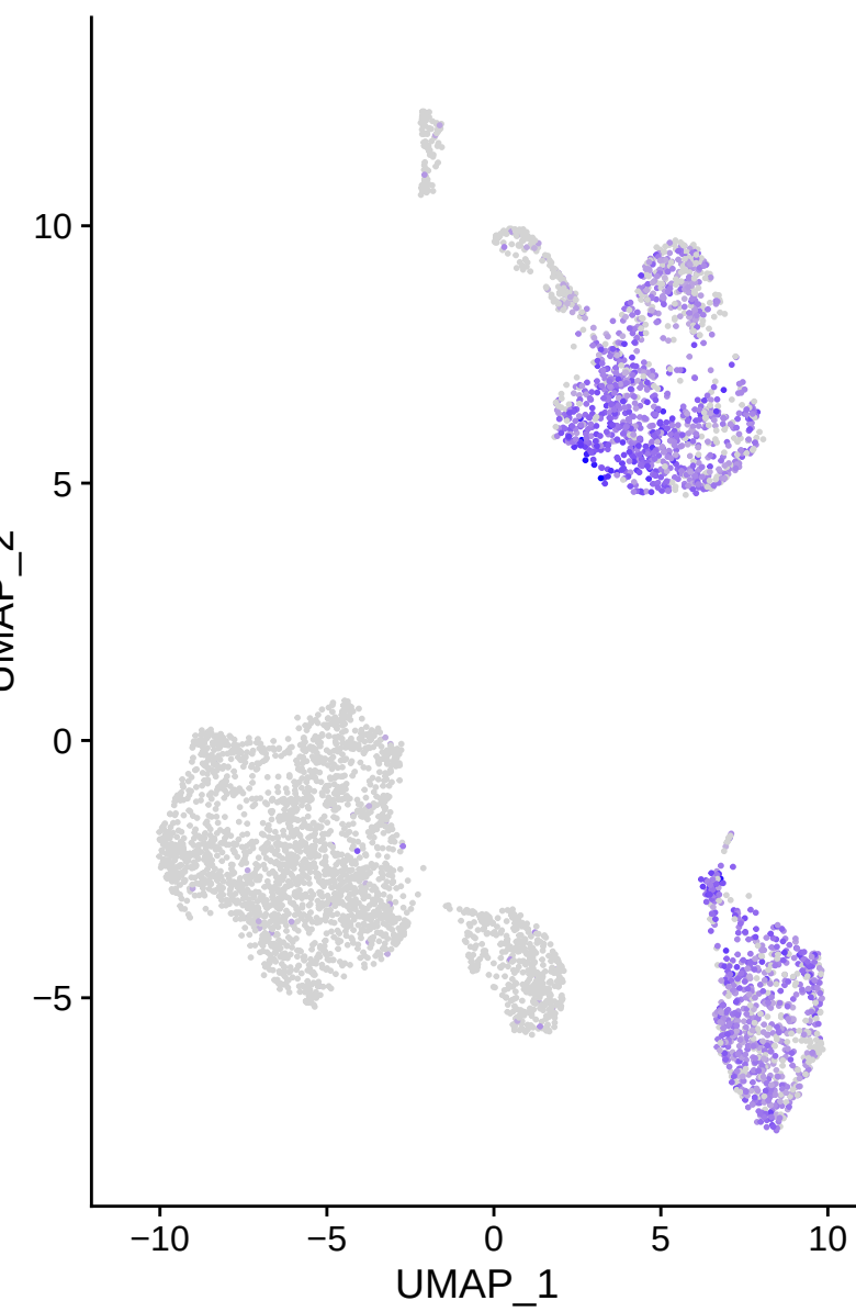
GATA3
