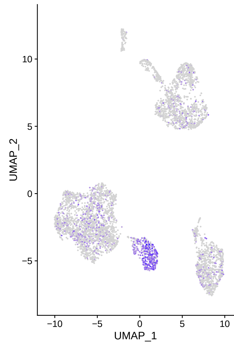
NANOG
