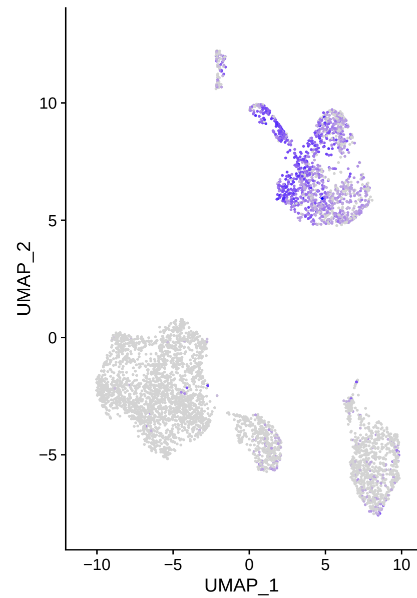
HAPLN1
