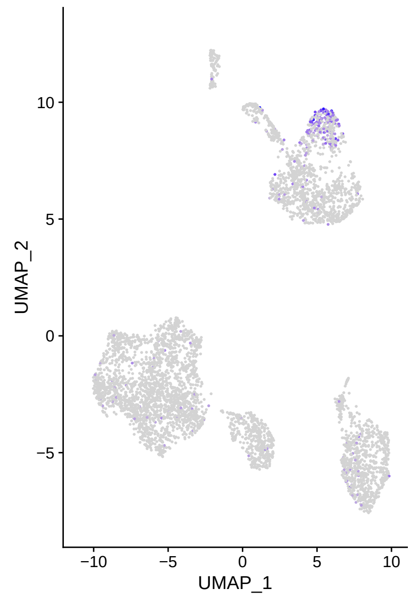
PAPPA2
