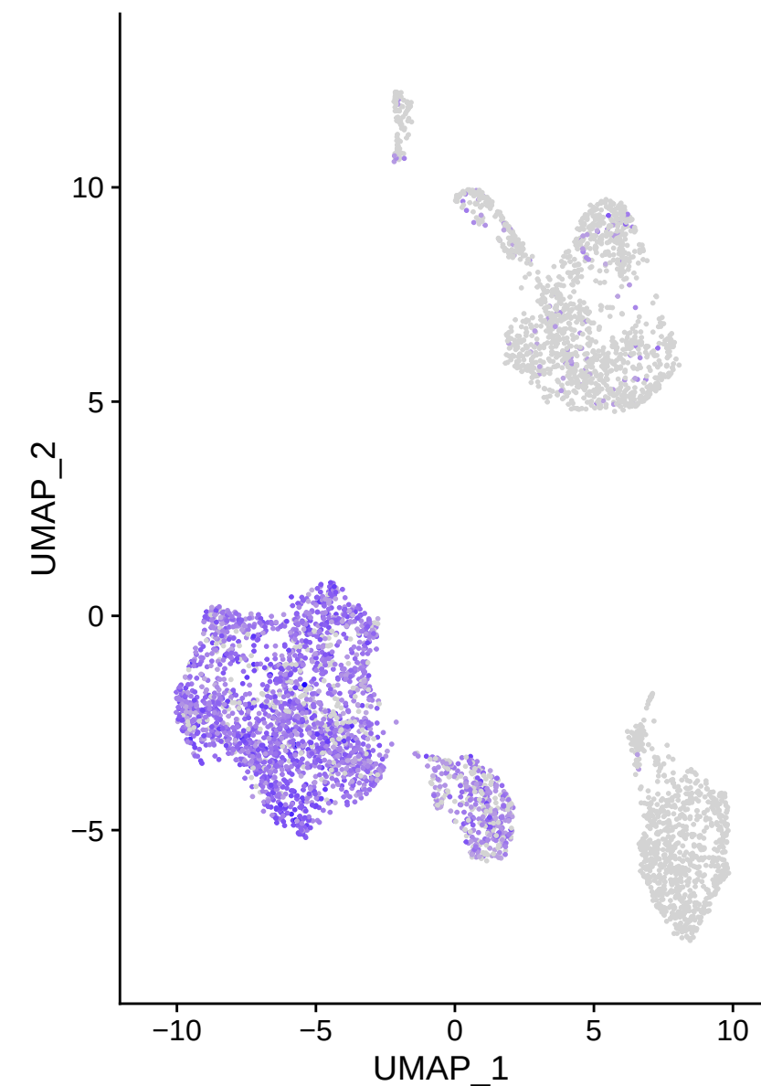
LIN28A
