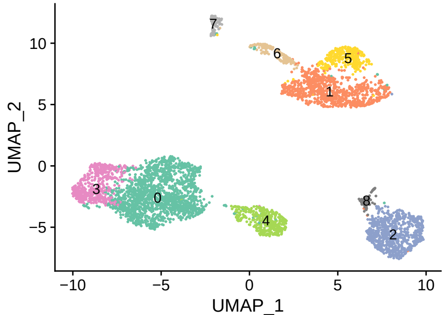
sf_snn_res.0.3
