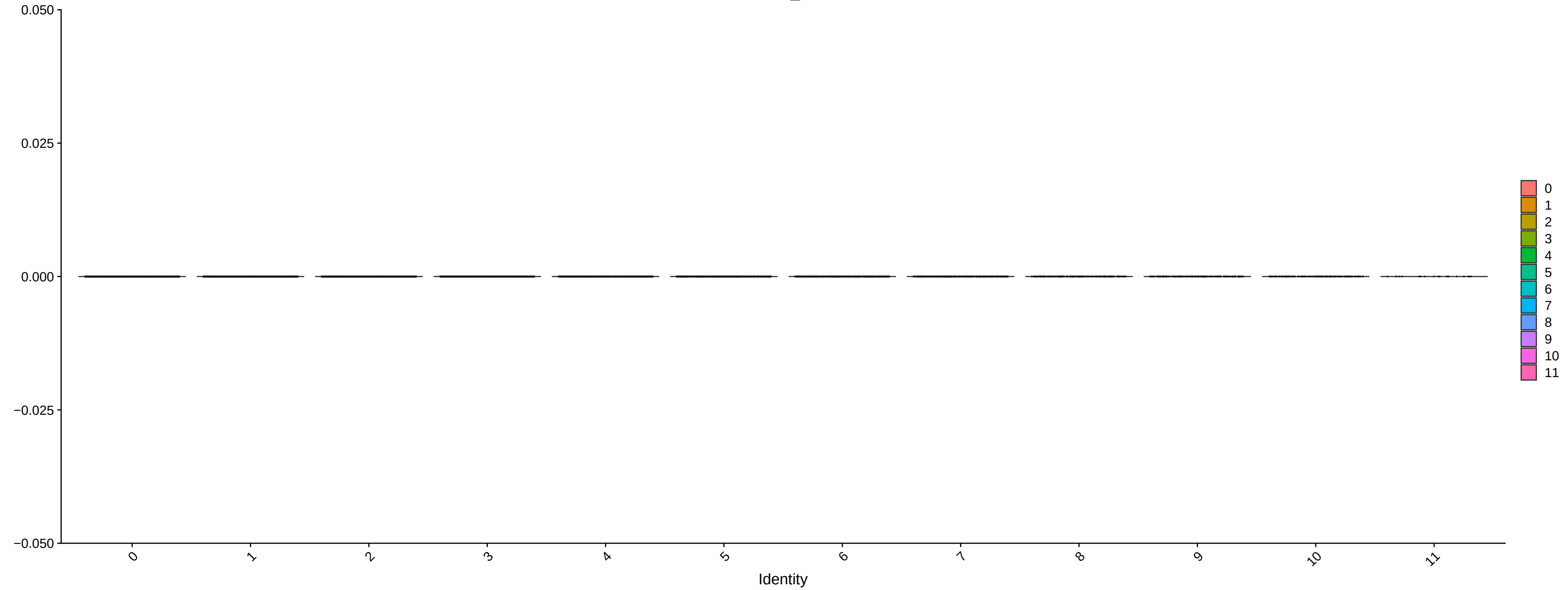
APC_A
