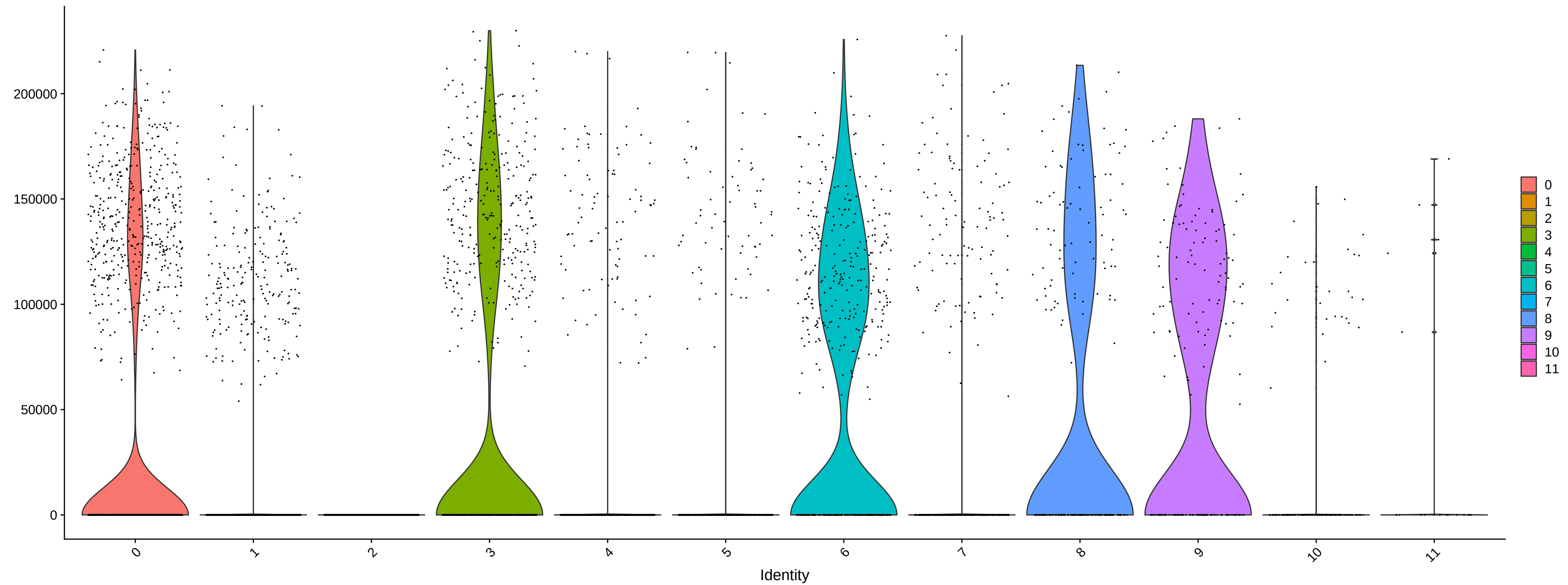
FSC_A
